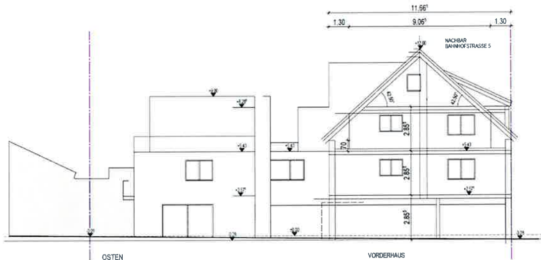
Schnitt
